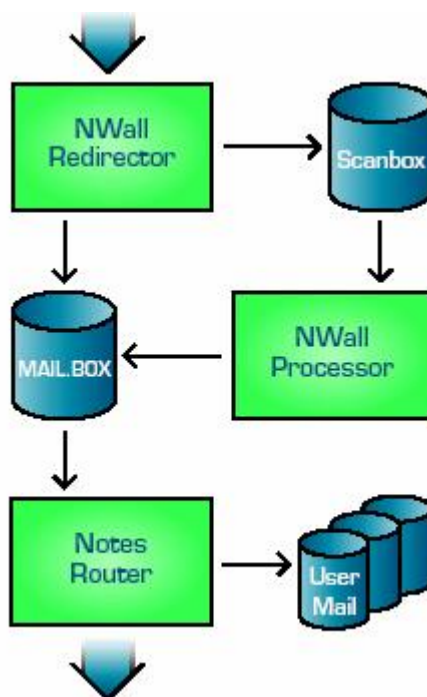
Obrázek 31 Schéma činnosti Lotus Notes & Domino [6].
