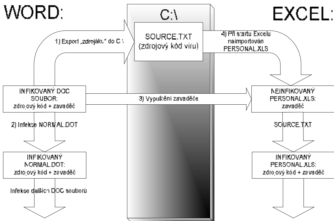
Obrázek 11 Princip fungování cross-infektorů, kdy je exportován zdrojový kód makroviru do speciálního souboru (v uvedeném případě SOURCE.TXT) a následně pak importován do dalších aplikací balíku Microsoft Office.
