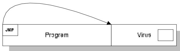
Obrázek 6 Schéma převzetí kontroly COM infektoru. Instrukce skoku JMP na samotném začátku předá řízení viru. V těle viru je zároveň uschován původní obsah oblasti, která byla nahrazena instrukcí skoku.
