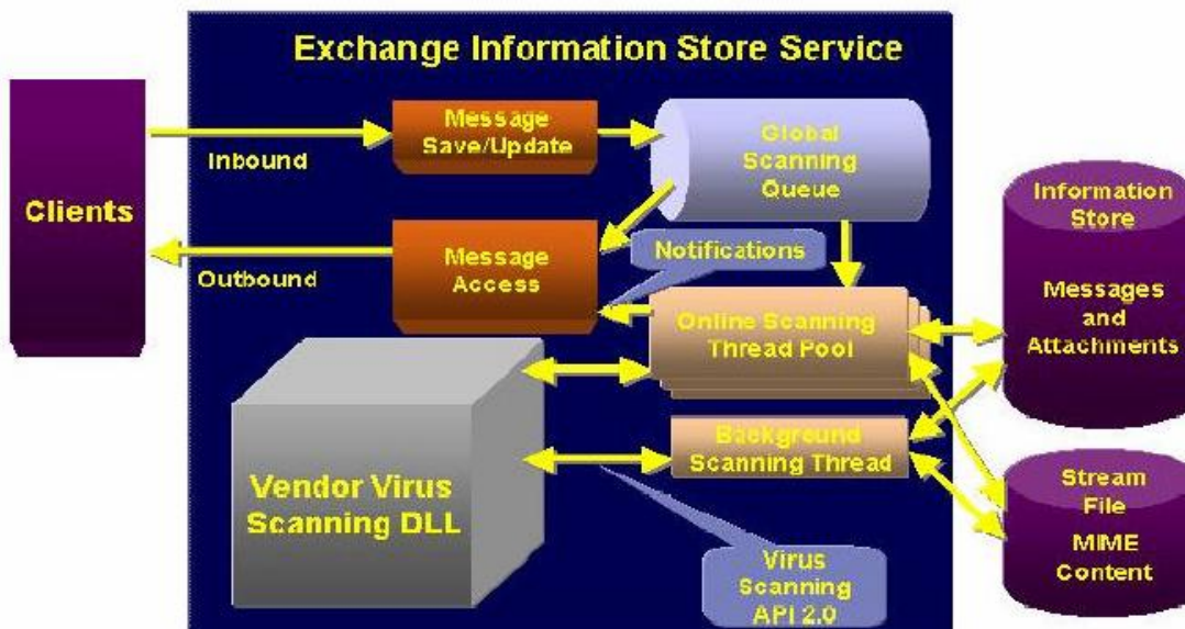
Obrázek 29 Rozhraní VSAPI 2.0 [6].
