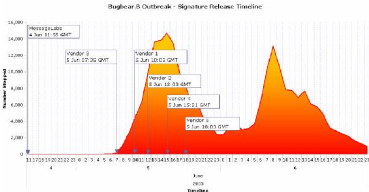
Obrázek 20 Virus Win32/BugBear.B.
