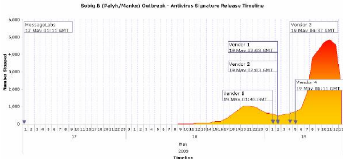
Obrázek 21 Virus Win32/Sobig.B.
