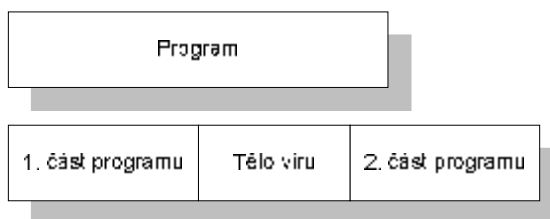
Obrázek 10 Metoda infekce – insert.
