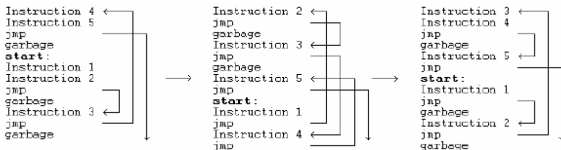
Obrázek 16 Tři různé generace viru Win95/Zperm [5].
