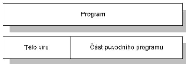
Obrázek 5 Přepisující virus (overwriting virus).
