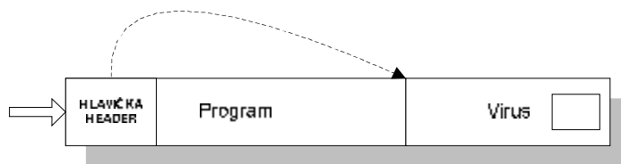
Obrázek 7 Schéma převzetí kontroly EXE infektoru. Hodnota entry pointu (CS:IP) v hlavičce ukazuje na kód viru.
