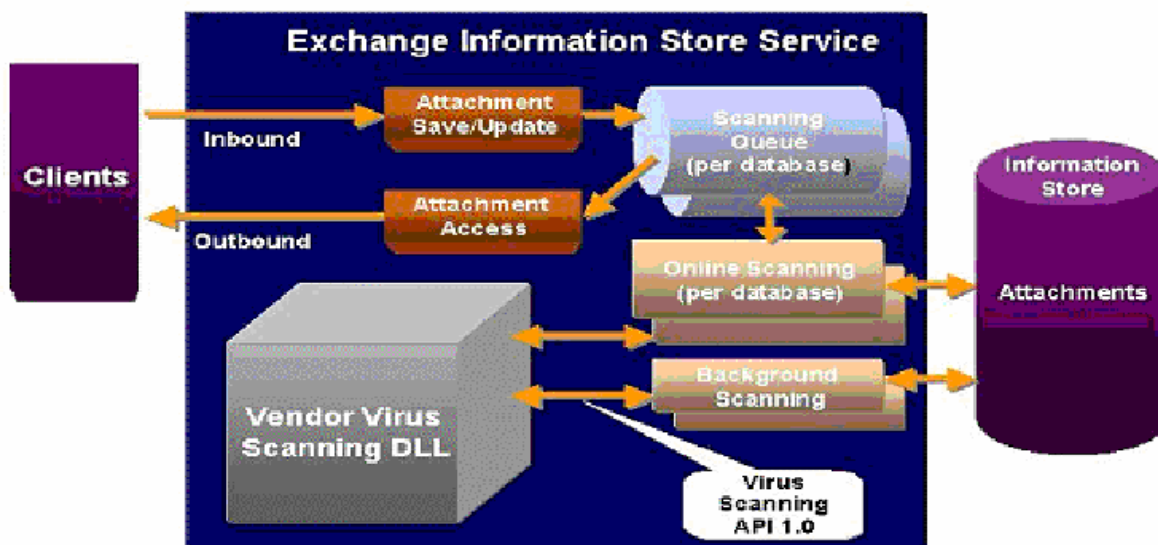
Obrázek 28 Rozhraní VSAPI 1.0 [6].
