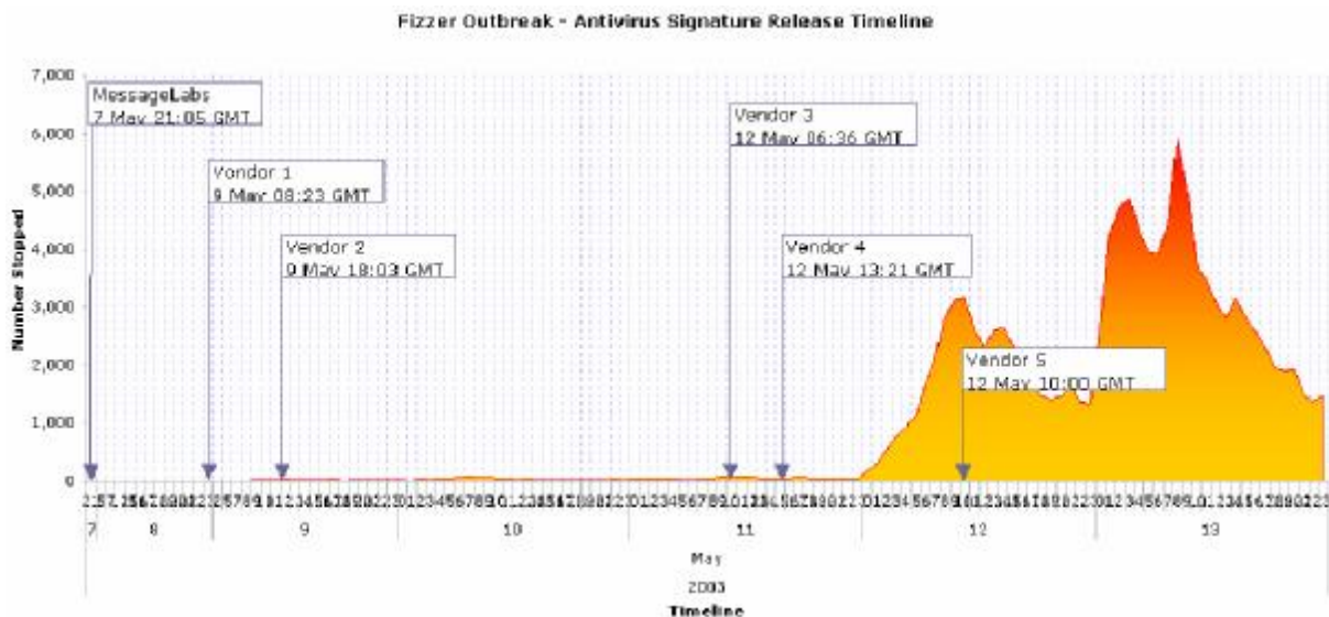
Obrázek 19 Virus Win32/Fizzer.A.
