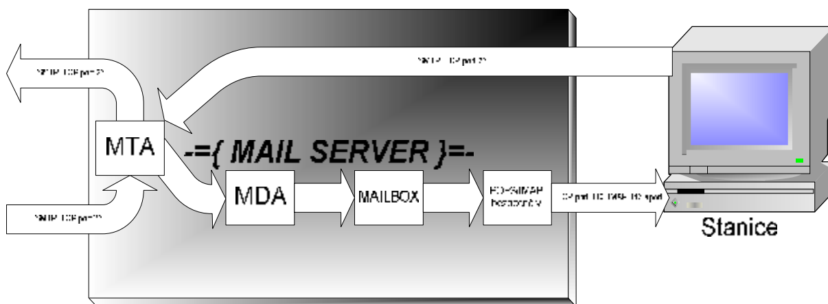
Obrázek 32 Schéma činnosti poštovního serveru pod Linuxem. MDA (Mail Delivery Agent) uloží e-mail do konkrétní schránky.
